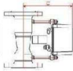
高温型 HT
