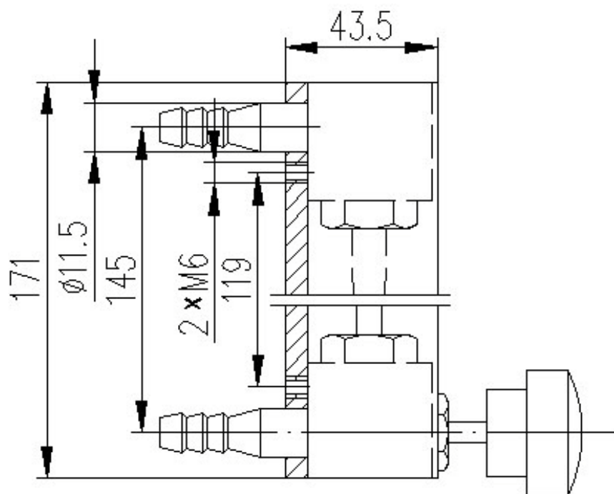
LZB-( )Q型流量计外形图
