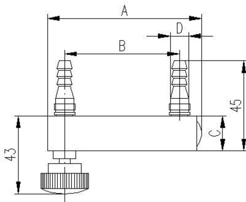
LZB-4M、6M型氧吧流量计外形图
