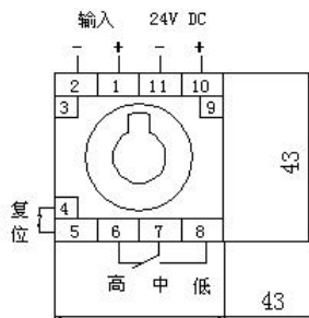
外形尺寸
