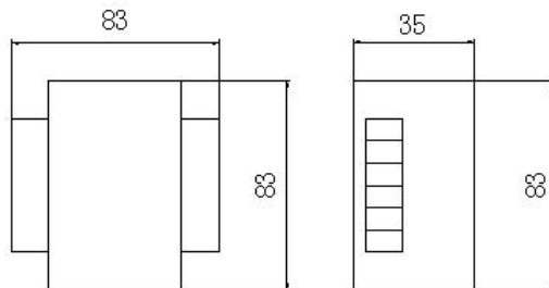
外形尺寸
