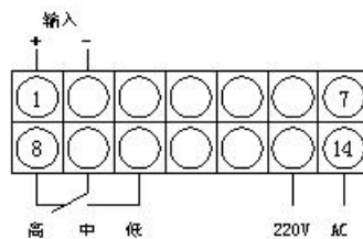
接线图
